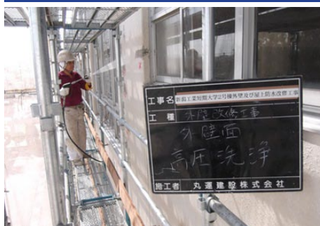
1) アロンウォール NEO 工法 高圧洗浄
