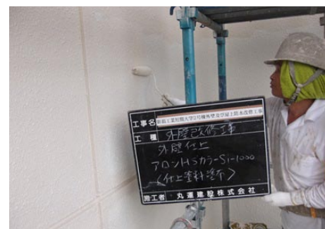
6) アロンウォール NEO 工法 アロンコート HS カラー Si-1000
