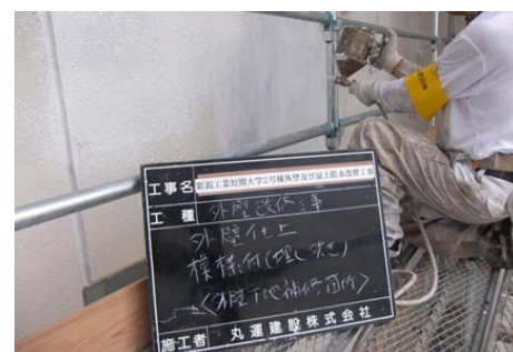
3) アロンウォール NEO 工法 模様付 (下地補修部分)
