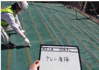
ケレン・清掃
