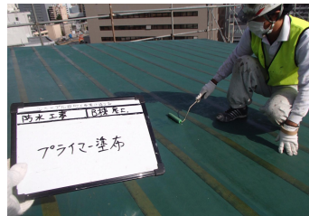
プライマー塗布
