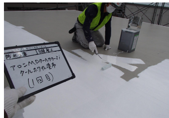
トップコート塗布
