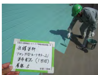
アロンMDルーフカラーS i 塗布状況 (1回目)
