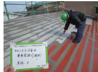
アロンコートSQ-H塗布状況 (1回目)
