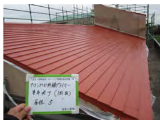
アロンMD防錆プライマー塗布完了
